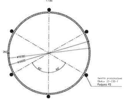
Rzut poziomu +227,50
