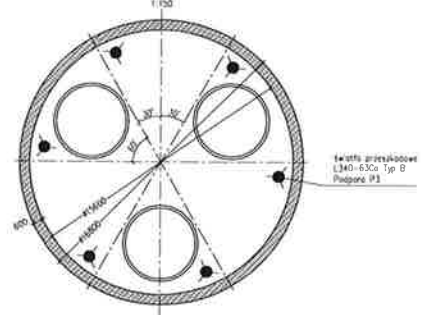
Rzut poziomu +257,50
