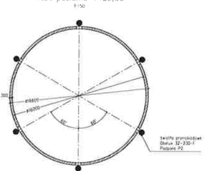
Rzut poziomu +182,50
