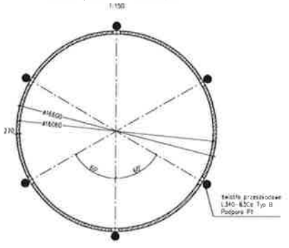
Rzut poziomu +182,50
