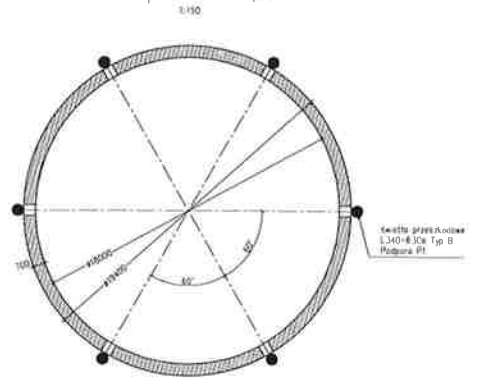
Rzut poziomu +47,50
