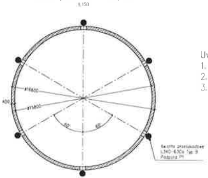
Rzut poziomu +137,50
