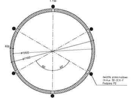
Rzut poziomu +92,50
