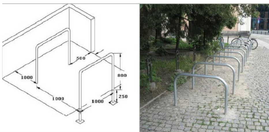
Ryc. 1. Stojaki rowerowe.
